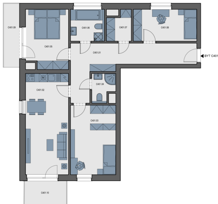
PŮDORYS PODLAŽÍ
